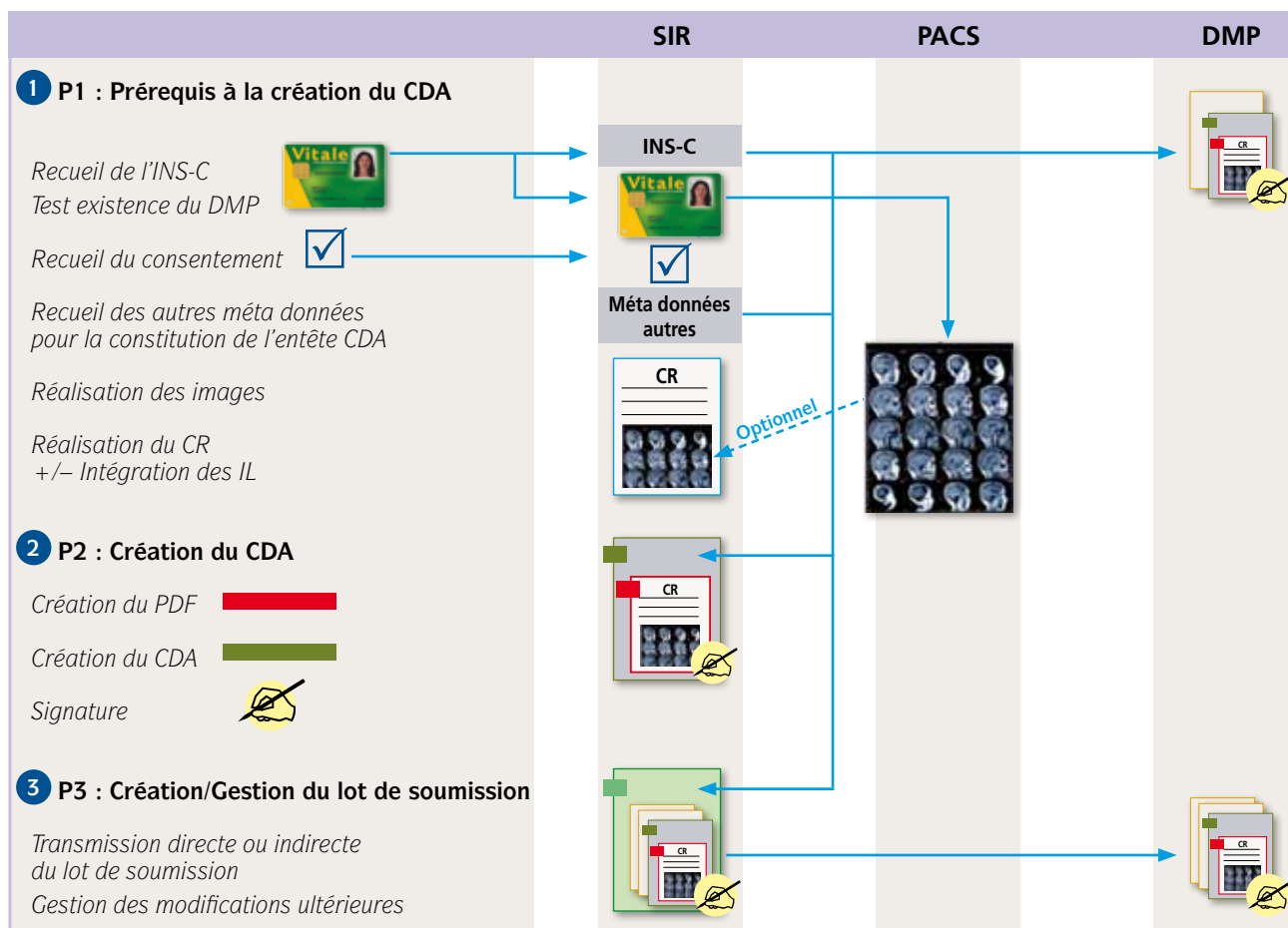
Figure 7.3.3-1 : Processus de création du CDA et du lot soumission. La gestion des images illustratives est facultative
